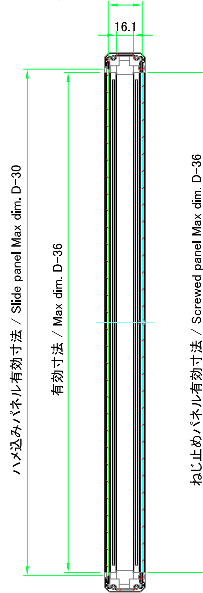
有効寸法 / Max dim. 31.5
